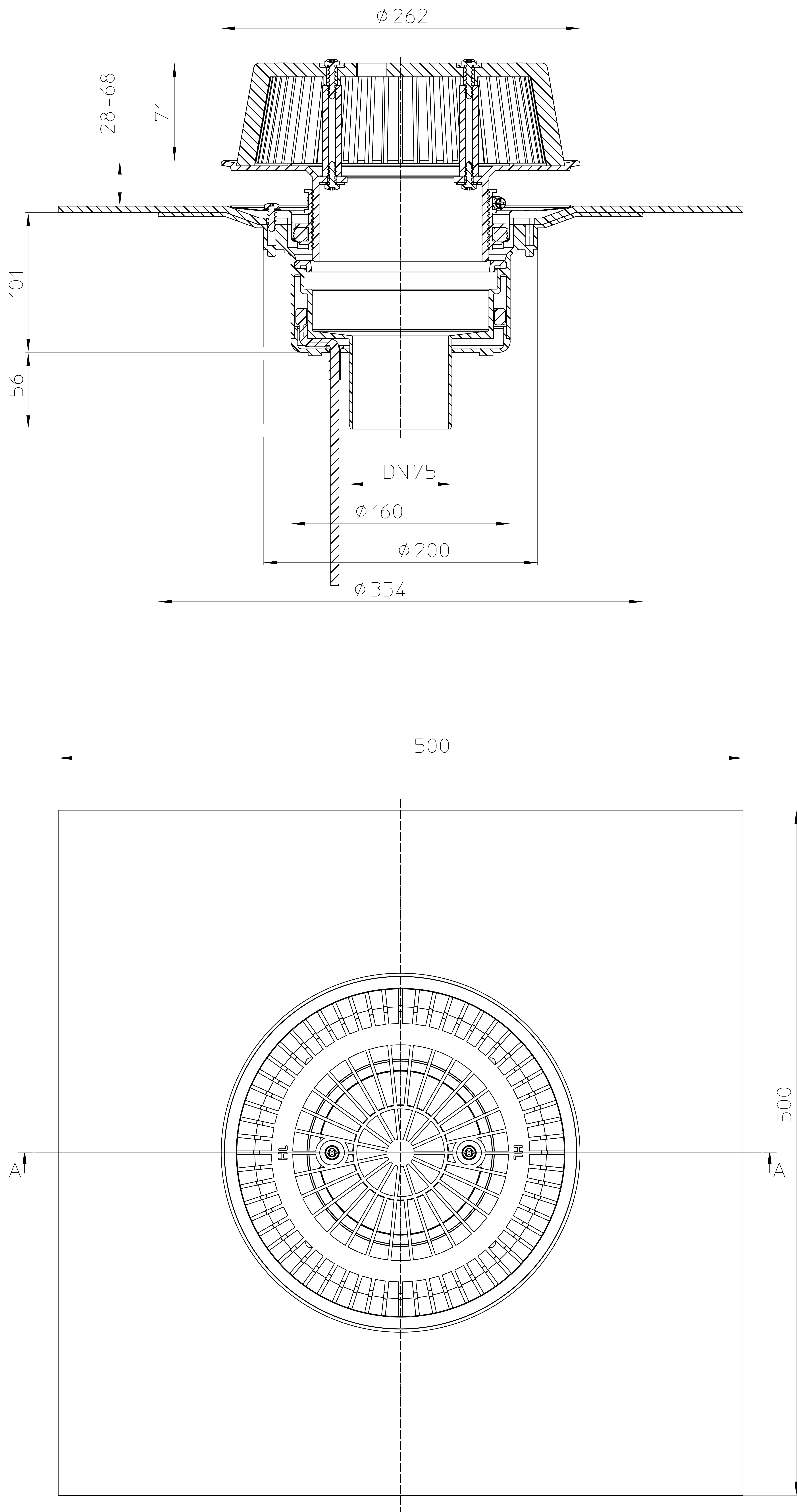
Schnitt A-A
